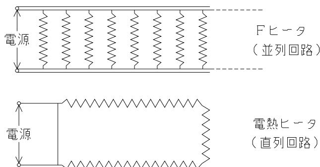
図 1 ヒートトレーサ (Fヒータ)の等価回路図
